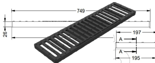
Grelha Sumidoura C250 FFD 750x200X27
