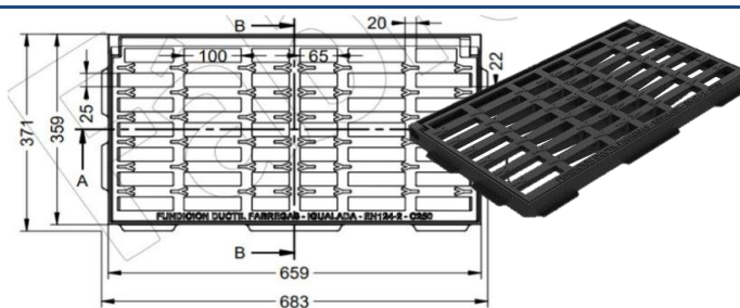
Grelha Sumidoura Anti-roubo C250 683x371x40 FAB.
