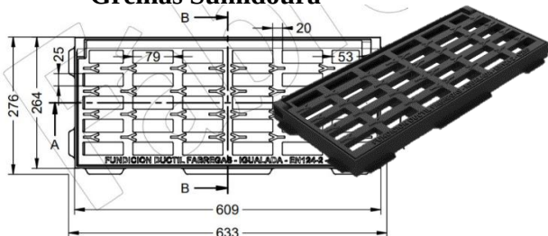
Grelha Sumidoura Anti-roubo C250 633x276x40 FAB.
